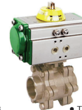
1/2"-2" 2000PSI
