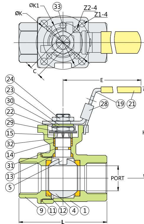
DIMENSIONS
