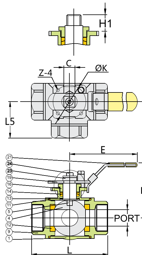
DIMENSIONS
